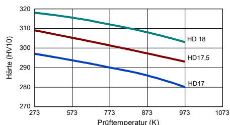
Warmhärte der HIGH-DENSITY Legierungen
